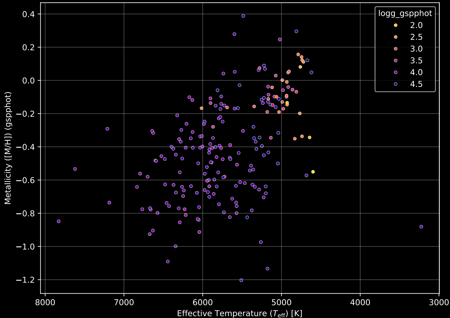
GALAH DR4 Field: [7239] Stellar Population Parameters (n= 202)
